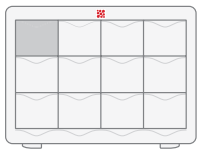
Tekli Çekmece: Tek Yükseklikli G 75 mm x Y 52 mm x D 223 mm
